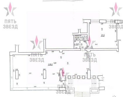
План 1 этажа Лиг. А
